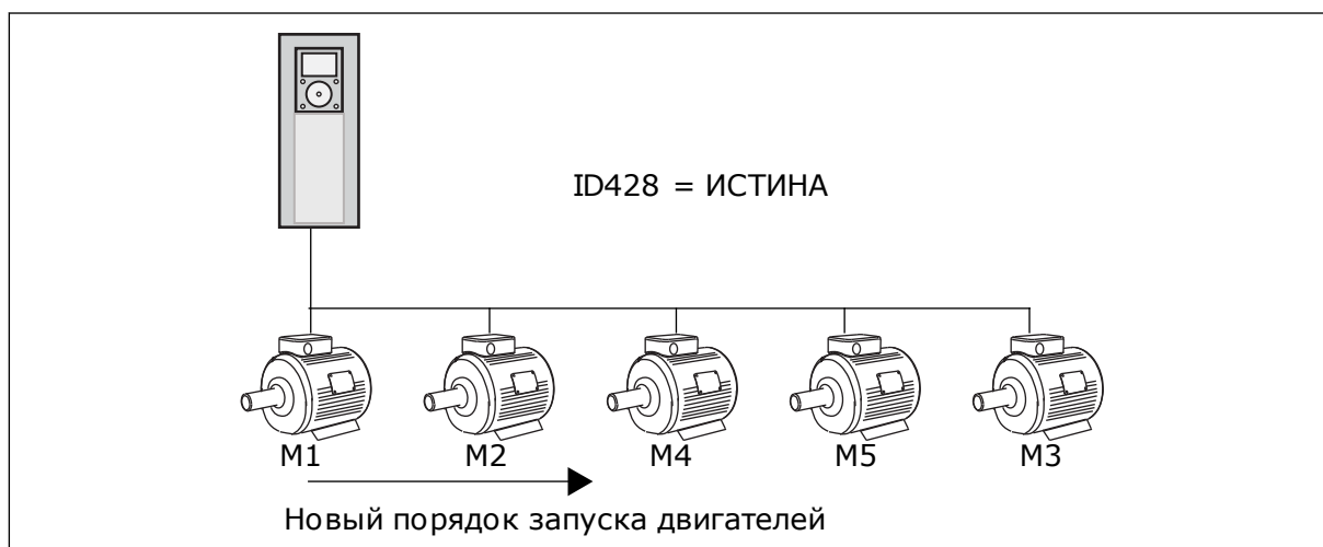
Рис. 82: Логика блокировки 3
