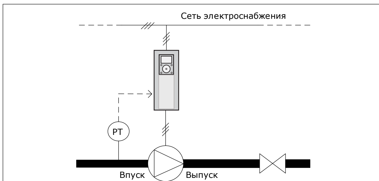
Рис. 85: Размещение датчика давления
