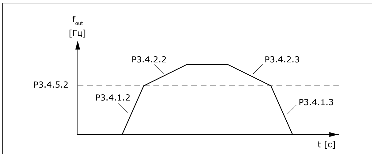
Рис. 49: Кривая 2 активируется, когда выходная частота превышает пороговый уровень. ( P3.4.5.2 = Пороговая частота кривой изменения скорости, P3.4.1.2 = Время разгона 1, P3.4.2.2 = Время разгона 2, P3.4.1.3 = Время замедления 1, P3.4.2.3 = Время замедления 2)
