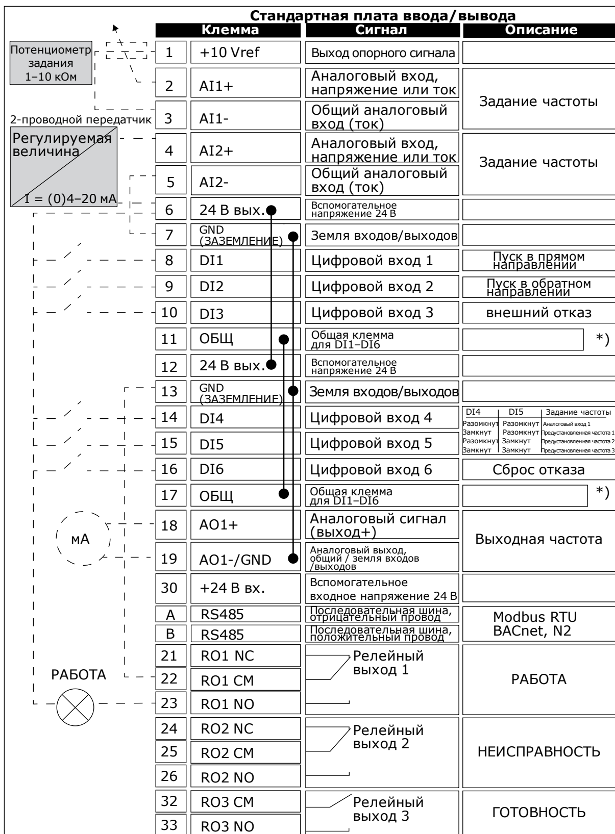
Рис. 39: Сигналы клемм управления привода на стандартной плате ввода/вывода и пример подключения. При заказе с дополнительным кодом +SBF4 релейный выход 3 замещается входом термистора.
