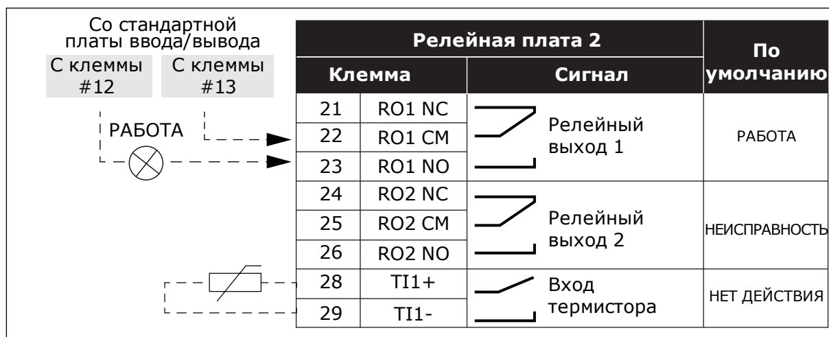
Рис. 41: Дополнительная релейная плата (+SBF4)
