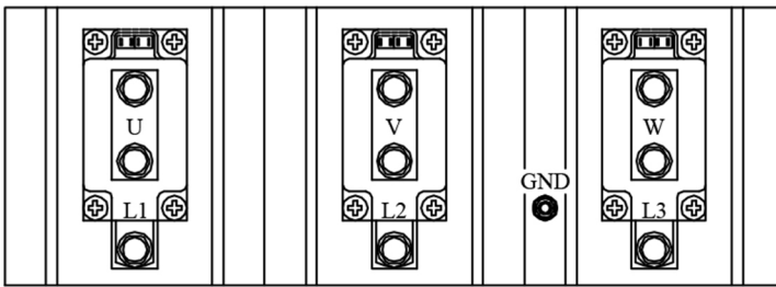
Силовые клеммы УПП СПРИНТ 45, 55, 75, 90, 100, 132, 160, 200, 225, 250.
