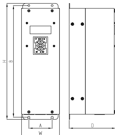
Рис. 2.3 Размеры УПП СПРИНТ 30, УПП СПРИНТ 37.
