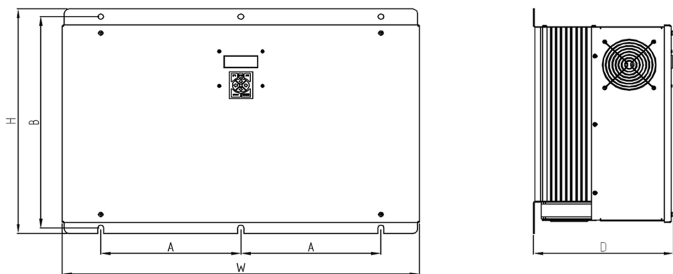
Рис. 2.8 Размеры УПП СПРИНТ 315, УПП СПРИНТ 400.
