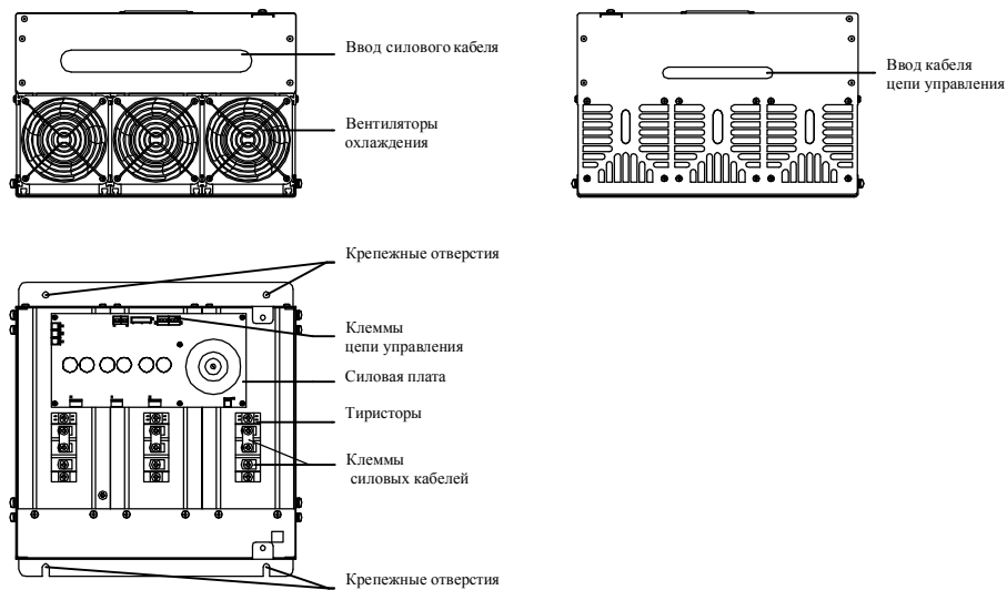
Рис.1.4 Составные части СПРИНТ 45, СПРИНТ 55, СПРИНТ 75.
