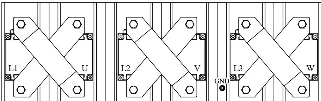
Силовые клеммы УПП СПРИНТ 315, 400.
