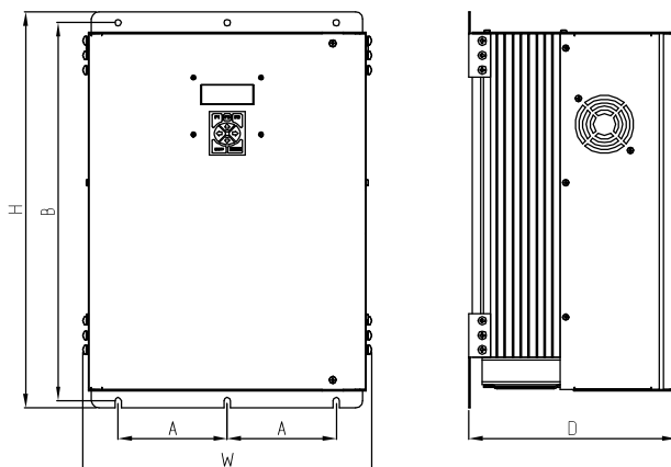
Рис. 2.5 Размеры УПП СПРИНТ 90, УПП СПРИНТ 110.
