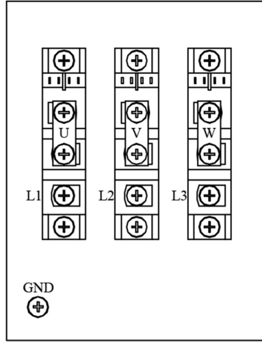
Силовые клеммы УПП СПРИНТ 7.5, 11, 15, 22, 30, 37.
