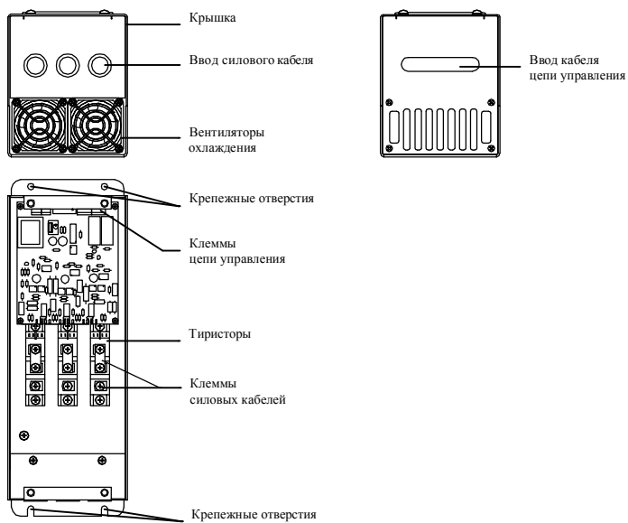
Рис.1.1 Составные части СПРИНТ 7.5, СПРИНТ 11.
