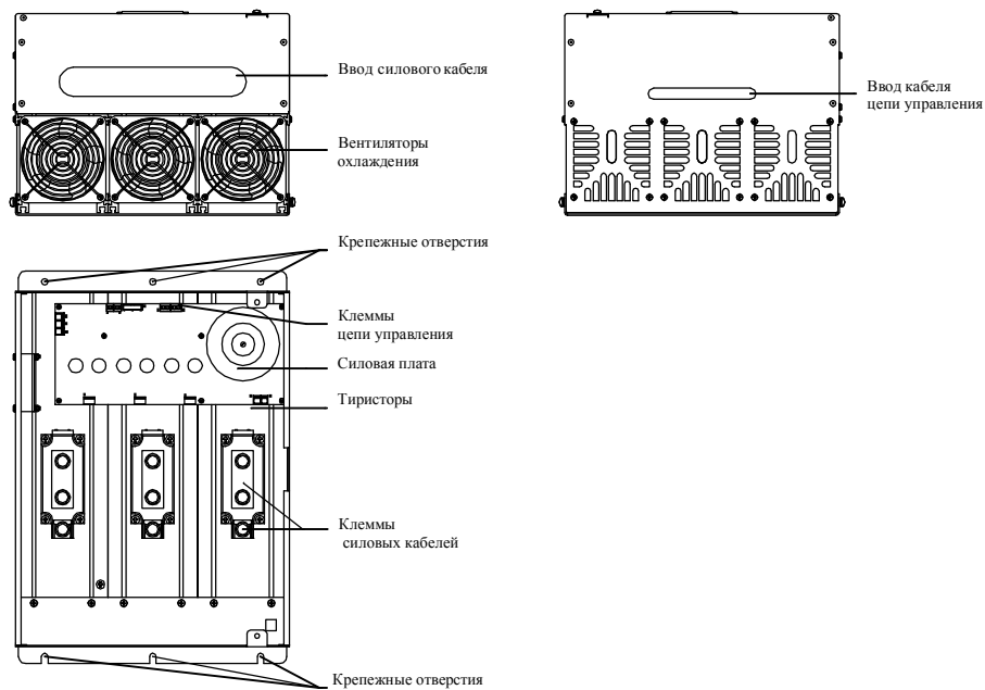
Рис.1.5 Составные части СПРИНТ 90, СПРИНТ 110.
