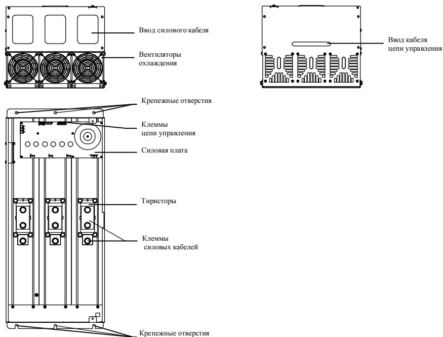
Рис.1.7 Составные части СПРИНТ 200, СПРИНТ 225, СПРИНТ 250.
