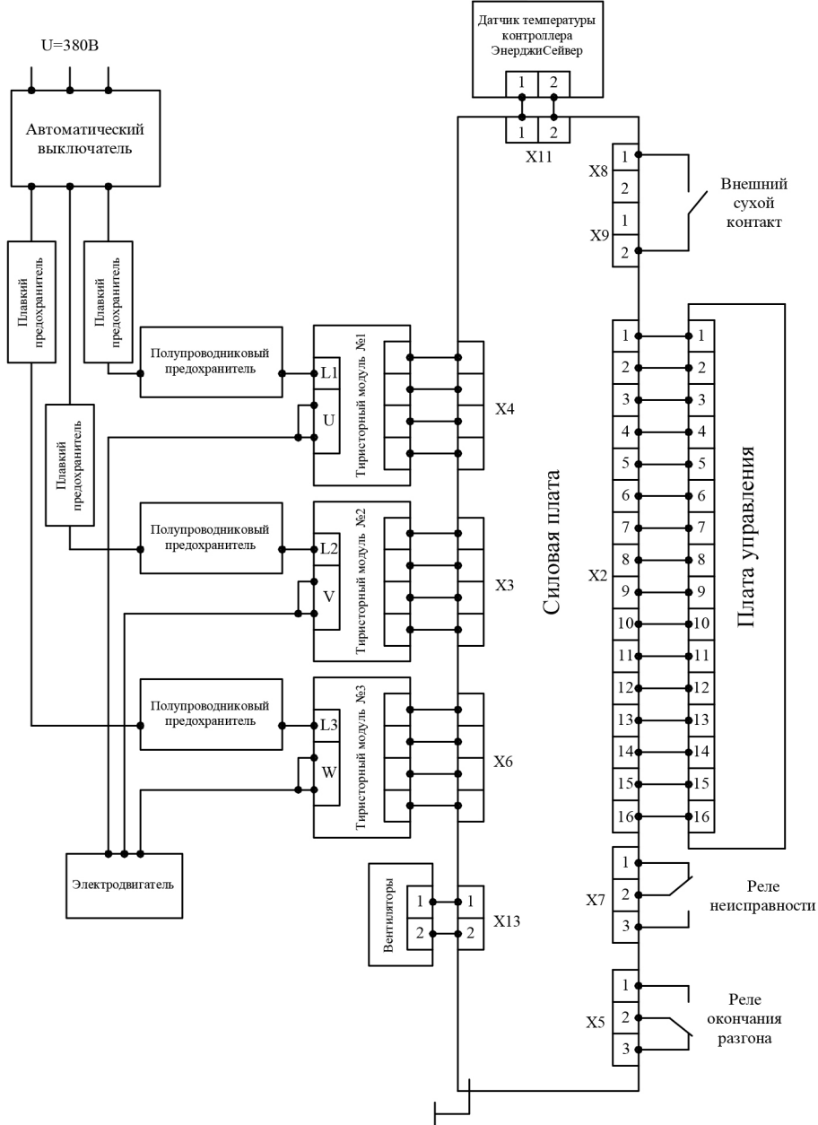
Рис.5.2 Общая схема подключения УПС СПРИНТ 45, 55, 75, 90, 110, 160, 200, 225, 250, 315, 400.
