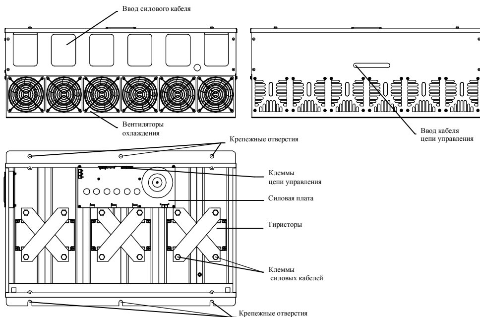
Рис.1.8 Составные части СПРИНТ 315, СПРИНТ 400.
