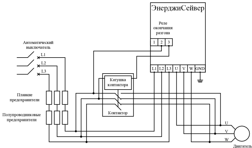
Рис.6.1 Подключение УПП СПРИНТ
