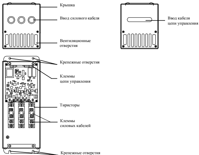
Рис.1.1 Составные части СПРИНТ 7.5, СПРИНТ 11.
