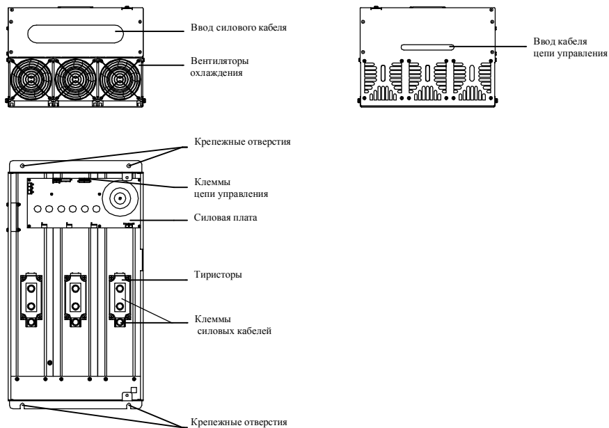
Рис.1.6 Составные части СПРИНТ 132, СПРИНТ 160.
