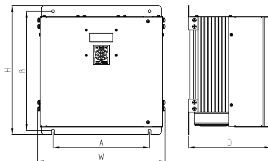
Рис. 2.4 Размеры УПП СПРИНТ 45, УПП СПРИНТ 55, УПП СПРИНТ 75 .
