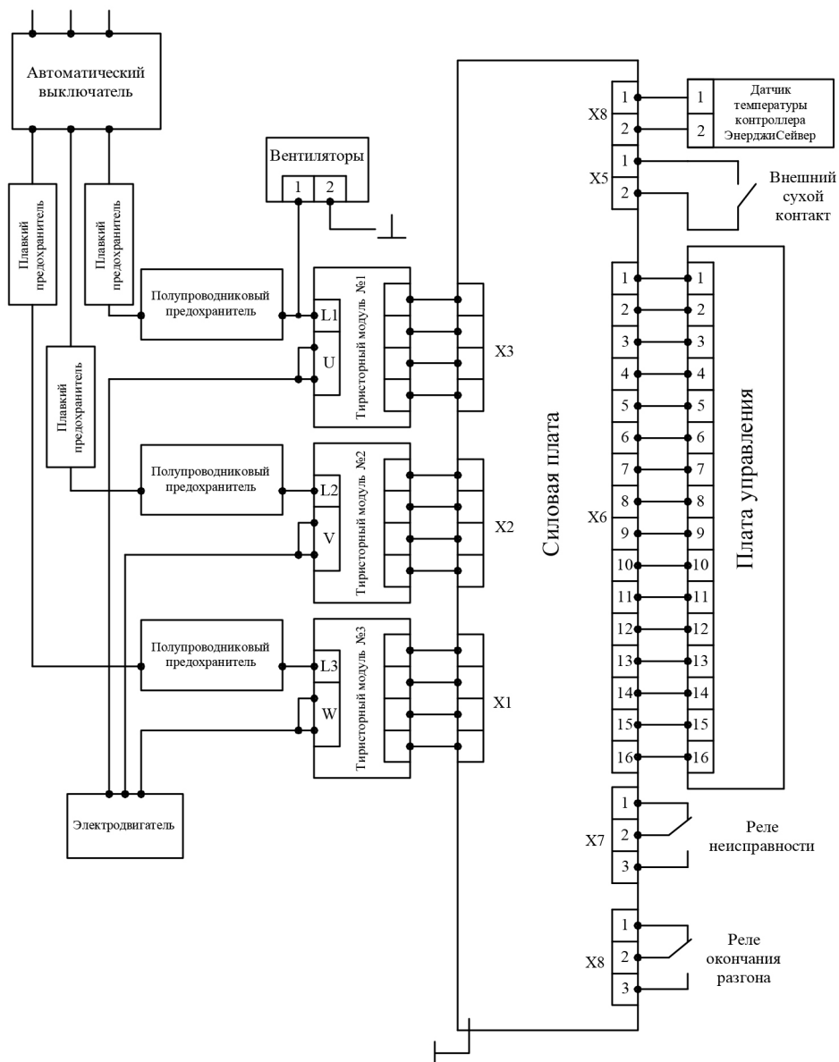
Рис.5.1 Общая схема подключения УПС СПРИНТ 7.5, 11, 15, 22, 30, 37.
