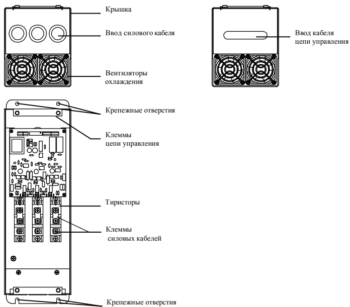
Рис.1.3 Составные части СПРИНТ 30, СПРИНТ 37.
