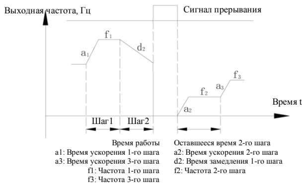
Рис.7-34 Режим перезапуска простого ПЛК 1
