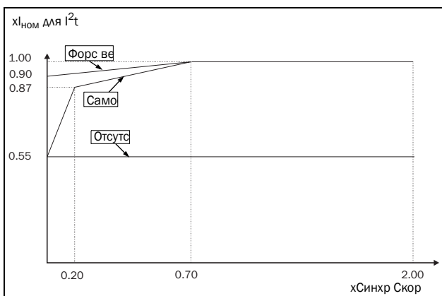
Рис. 76 Кривые I 2 t
