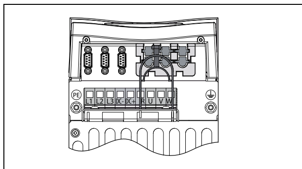
Рис. 11 Вид снизу, устройство Emotron VFX моделей 48-025 – 48-045 (типоразмер корпуса C2), с кабельным интерфейсом для подключения электрической сети, электродвигателя, опции DC+/DC-, тормозного резистора и управления
