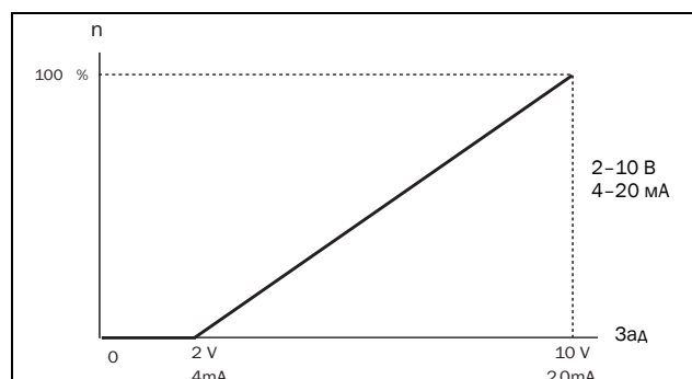
Рис. 109 2-10 В/4-20 мА (реальный ноль)
