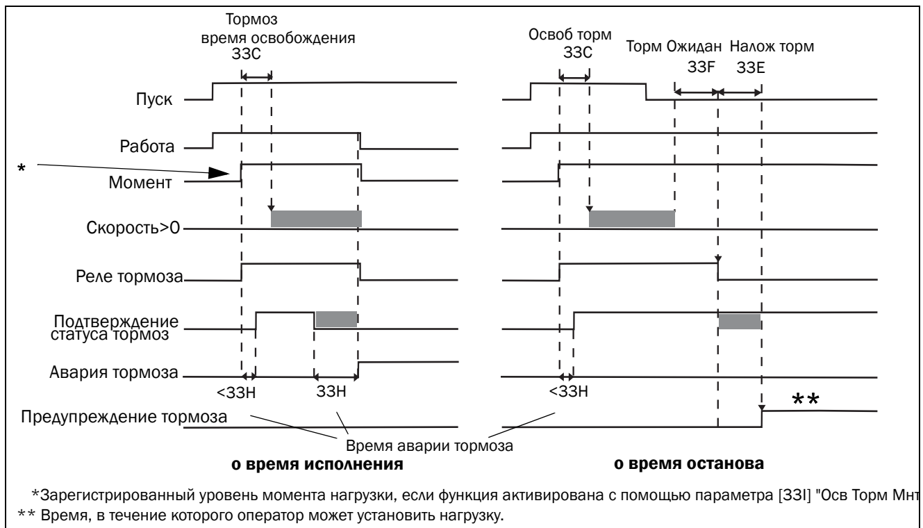
Рис. 86 Принцип работы тормоза при аварии в процессе исполнения и во время останова
