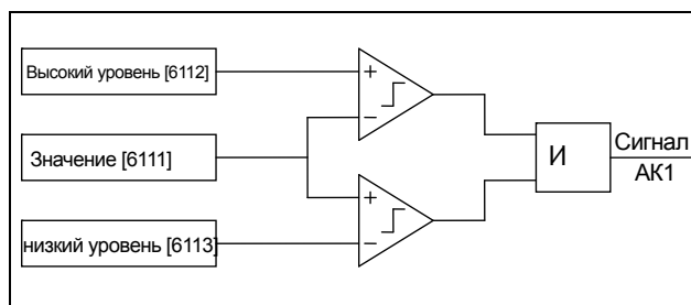
Рис. 114 Аналоговый компаратор двухпорогового типа
