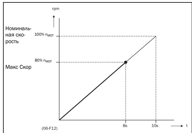
Рис. 80 Время разгона и максимальная скорость
