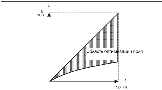
Рис. 91 Оптимизация поля
