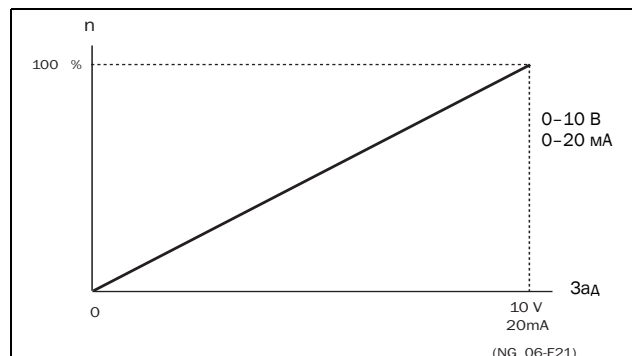
Рис. 108 Обычная конфигурация во всем диапазоне
