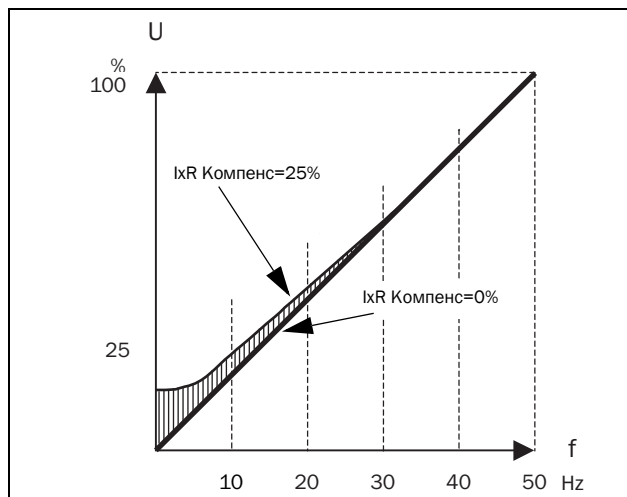
Рис. 90 IxR компенсация при линейной зависимости В/Гц
